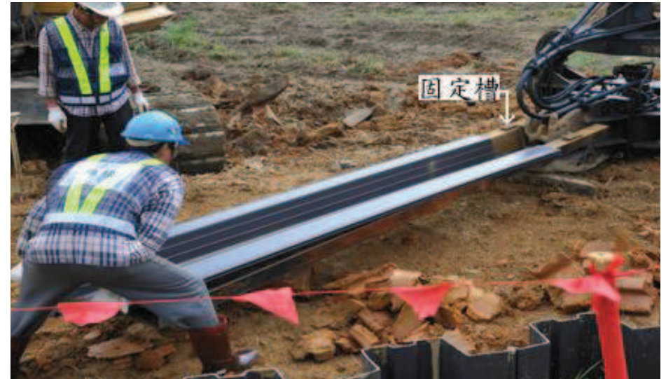
步驟四：底部以U型夾固定
